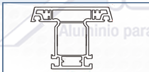
Contramarco Doble Ventana Abatible ( P60-ST(D) )
