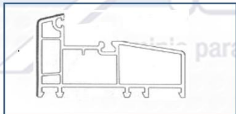
Contramarco Vidrio Fijo 80mm (T80-GDKD)
