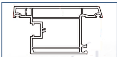
Hoja Hacia Fuera Puerta Abatible ( P60-MS)
