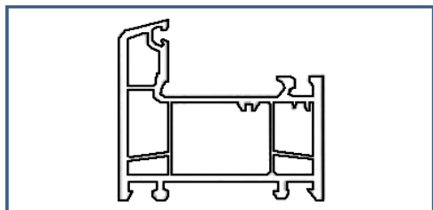
Contramarco Ventana Abatible ( P60-K(D) )
