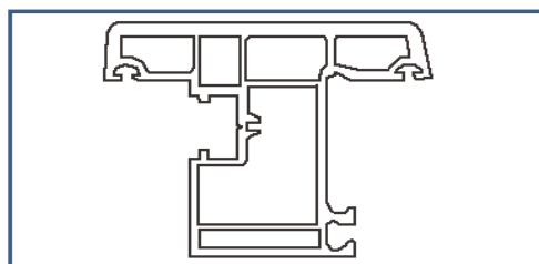
Hoja hacia afuera Ventana Abatible (P60-WKS)
