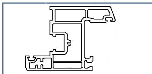
Hoja hacia dentro Ventana Abatible (P60-NKS)
