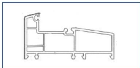
Contramarco Vidrio Fijo 88mm (T88-GDK)
